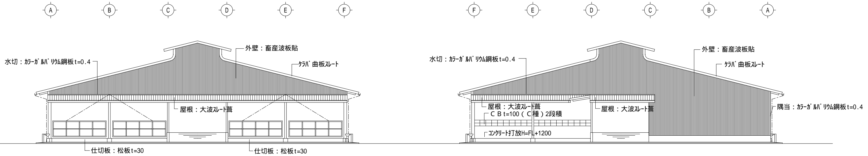
1 立面図 S=1/150
