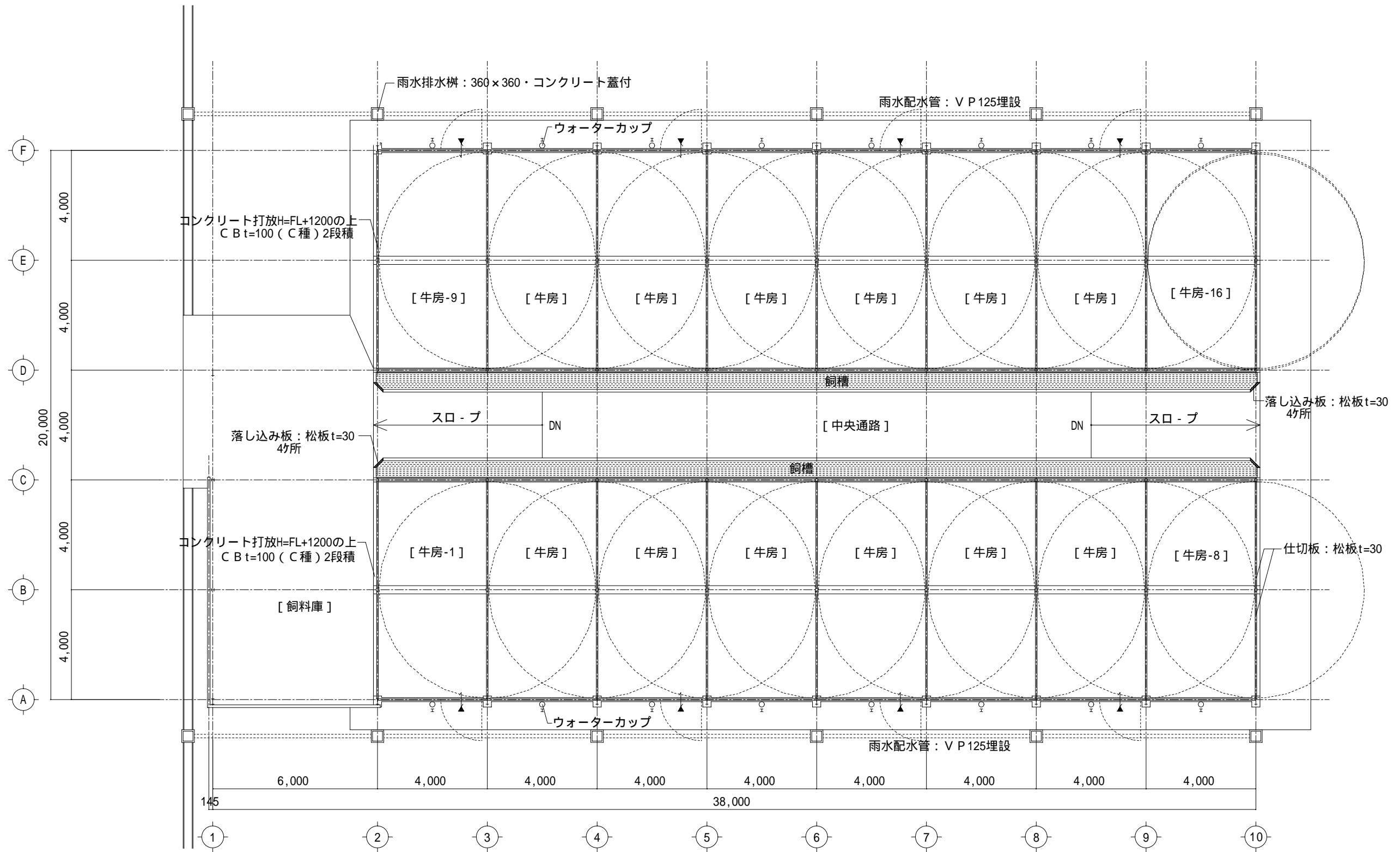
平面図 S=1/150
