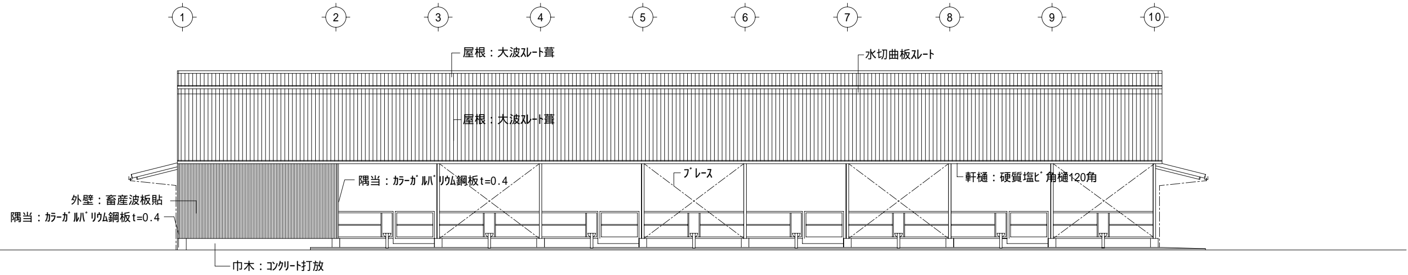
A 立面図 S=1/150
