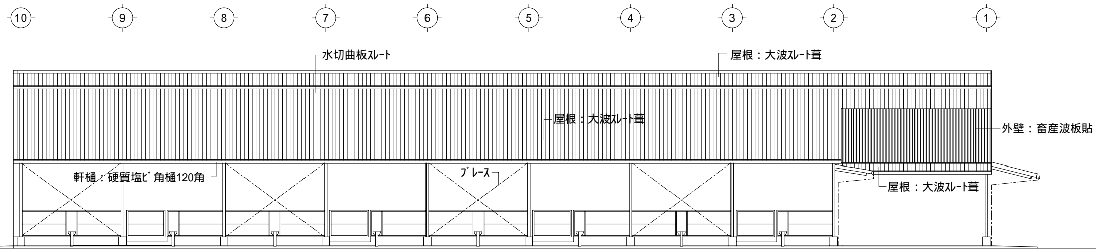
1 立面図 S=1/150
