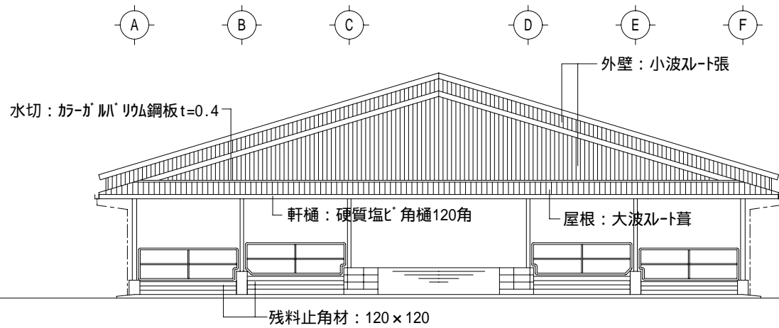
1 2 立面図 S=1/150
