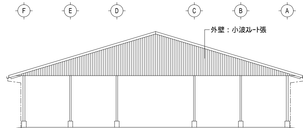
1 立面図 S=1/150
