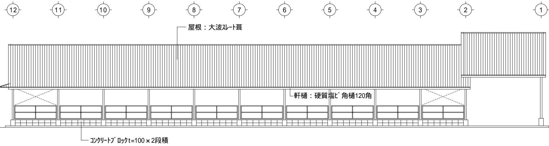
F 立面図 S=1/150
