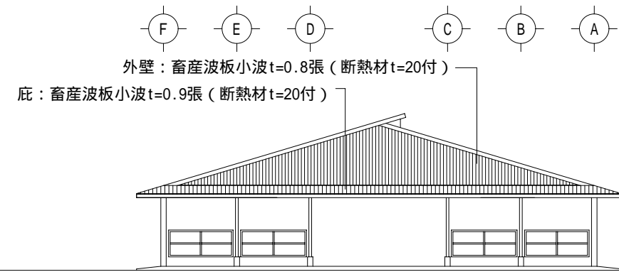
1 立面図 S=1/200
