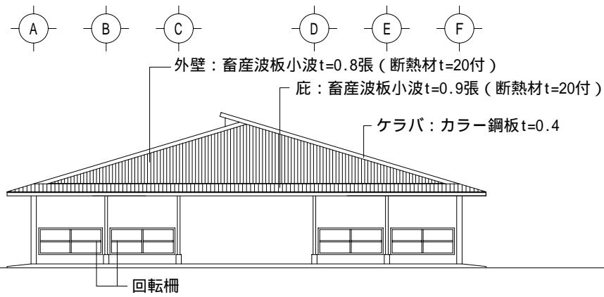
1 3 立面図 S=1/200
