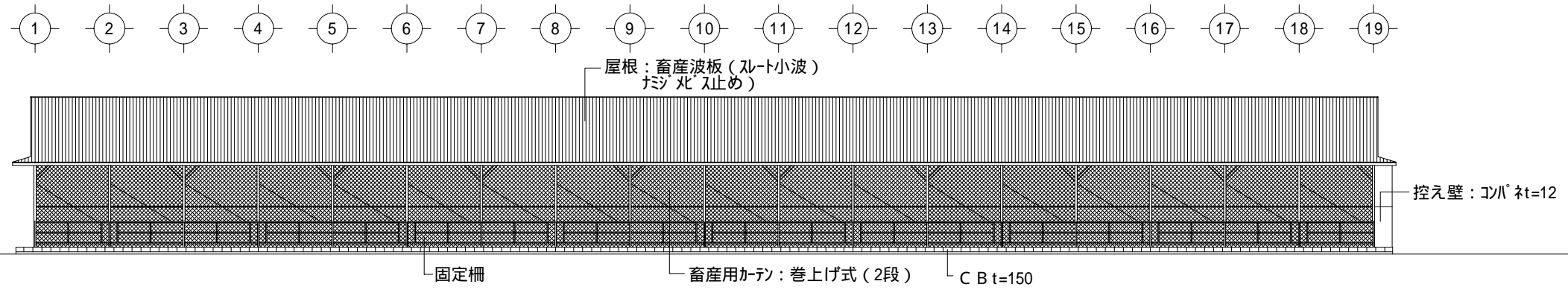
A 立面図 S=1/250
