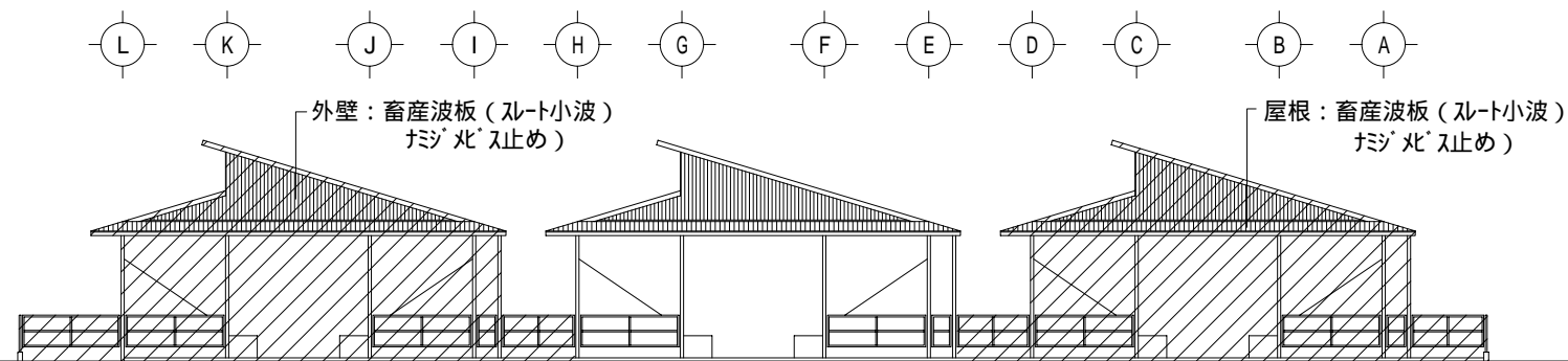
1 立面図 S=1/250
