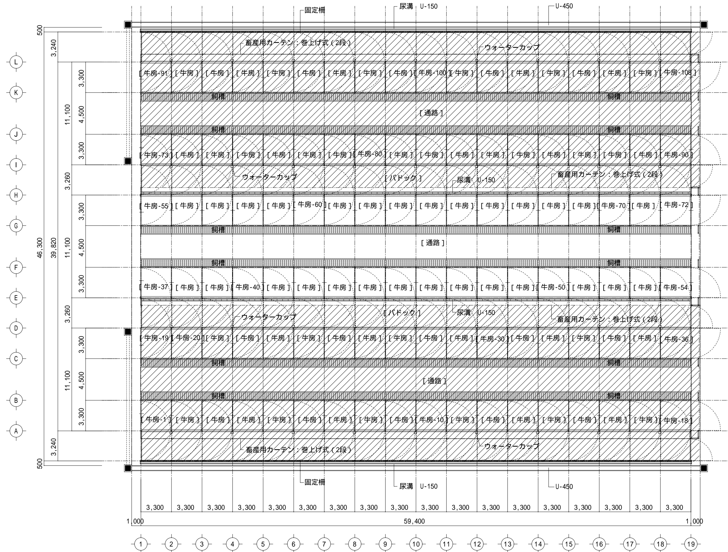
平面図 S=1/200
