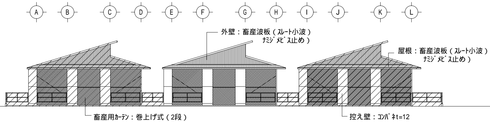
19 立面図 S=1/250
