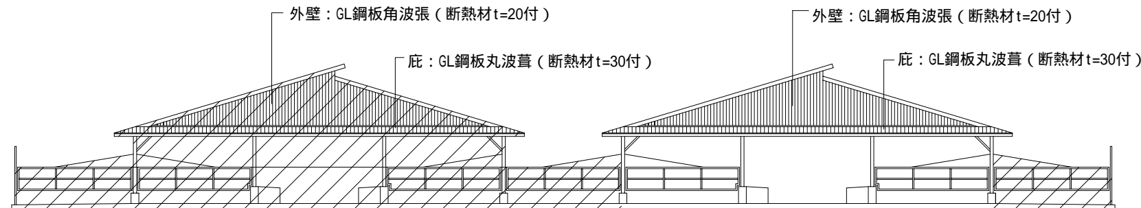
1・13立面図 S=1/200
