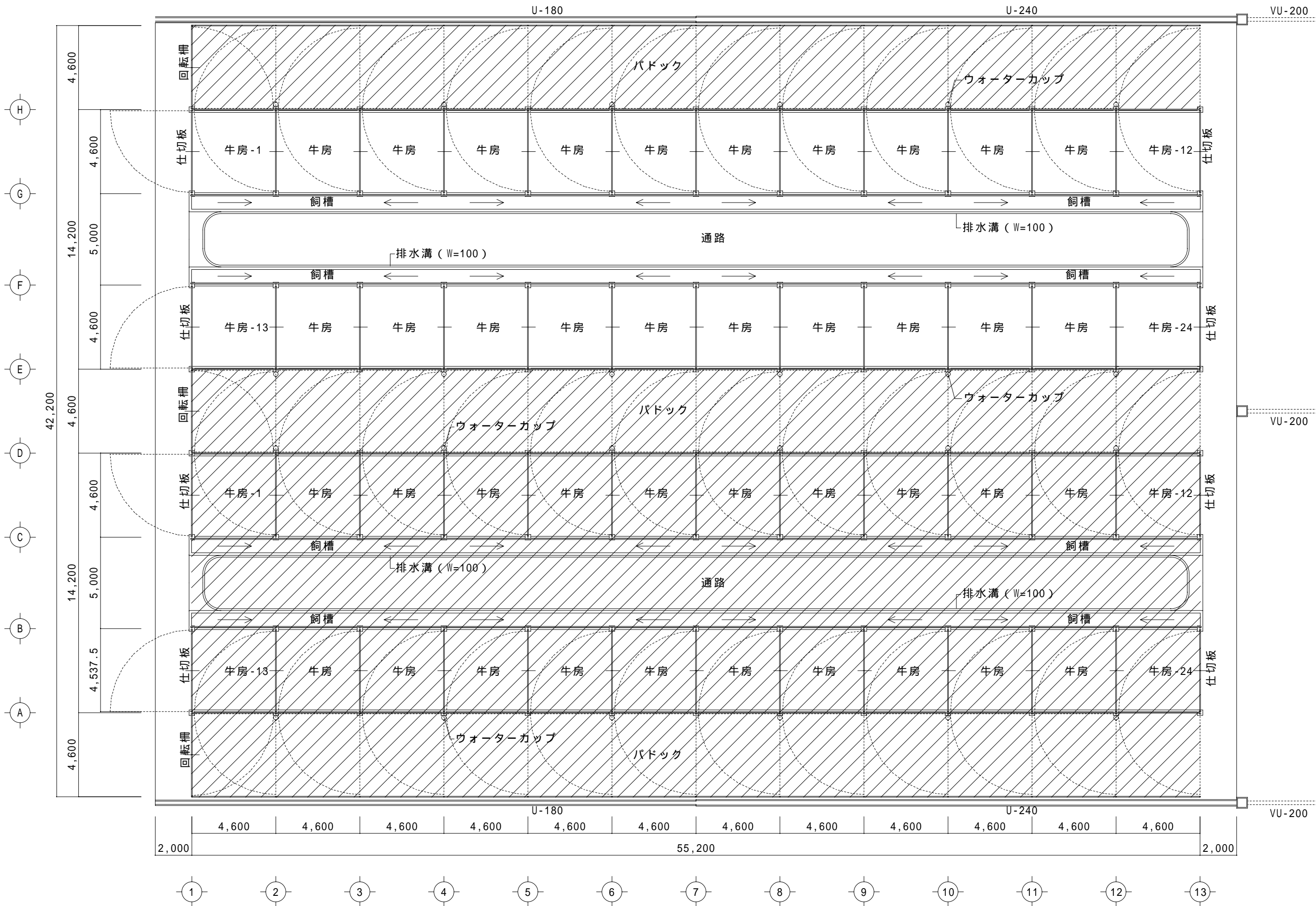
平面図 S=1/200
