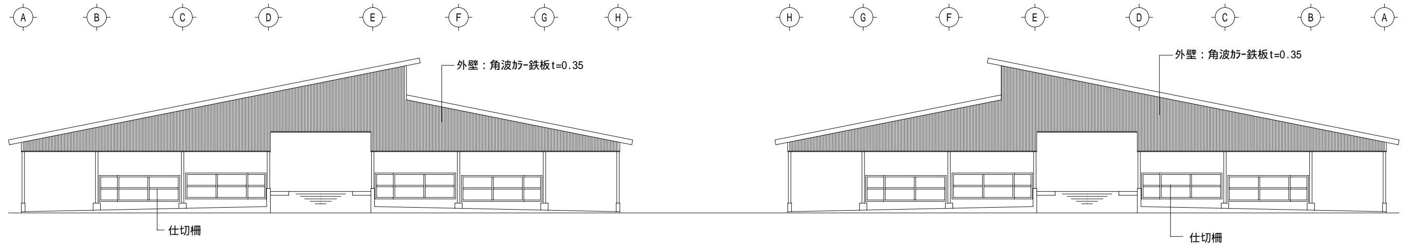
1 立面図 S=1/150
