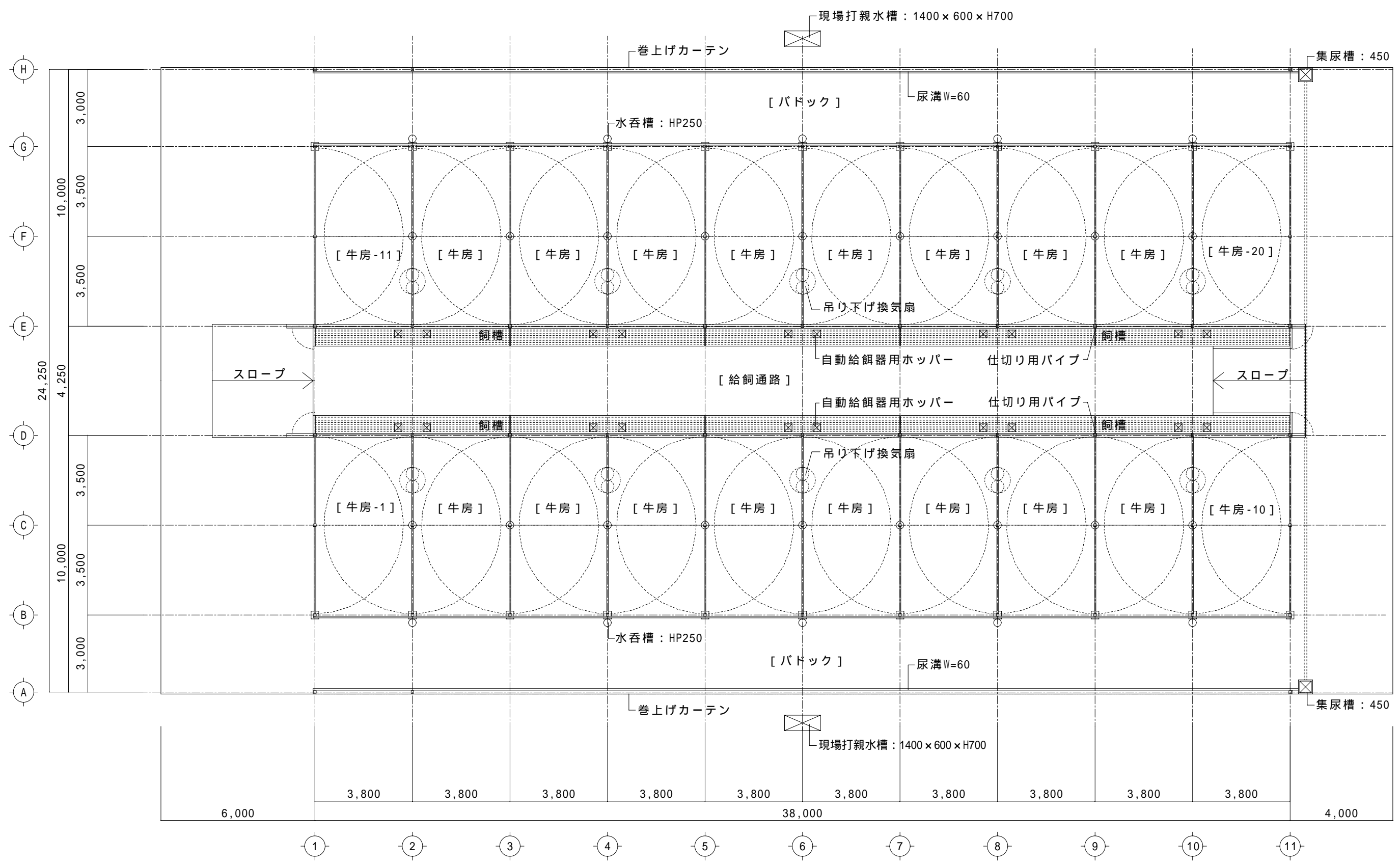
平面図 S=1/150
