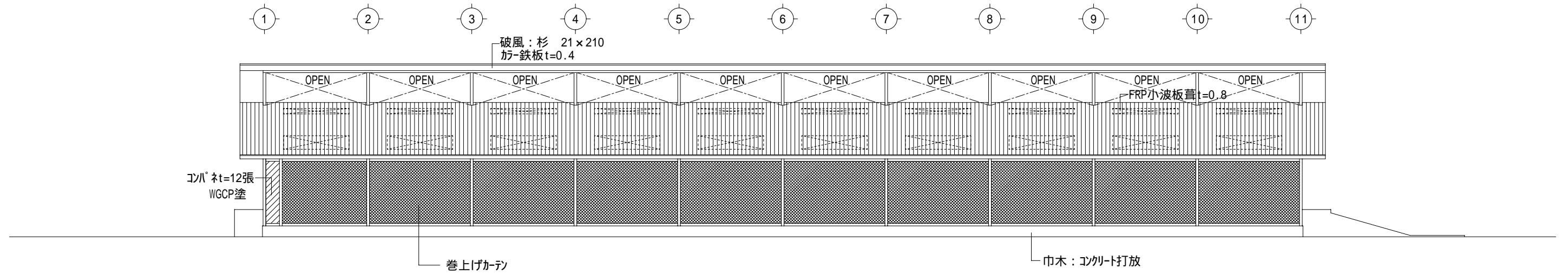
A 立面図 S=1/150
