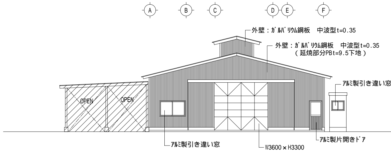
A 立面図 S=1/150
