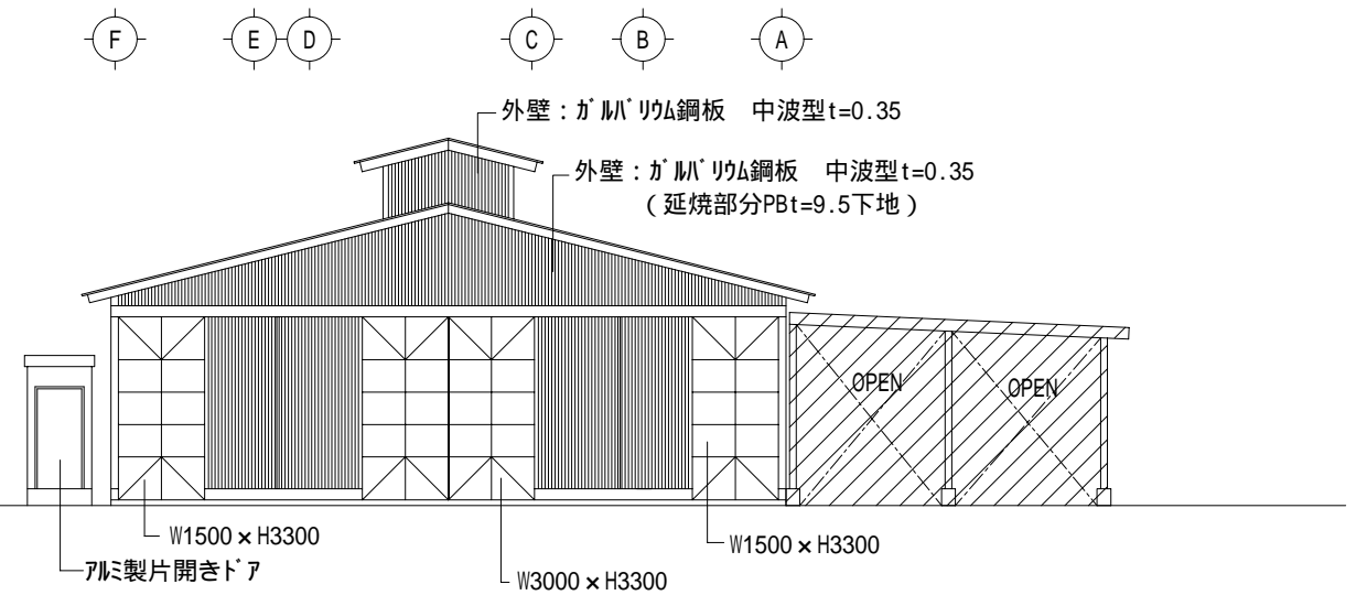
1 立面図 S=1/150
