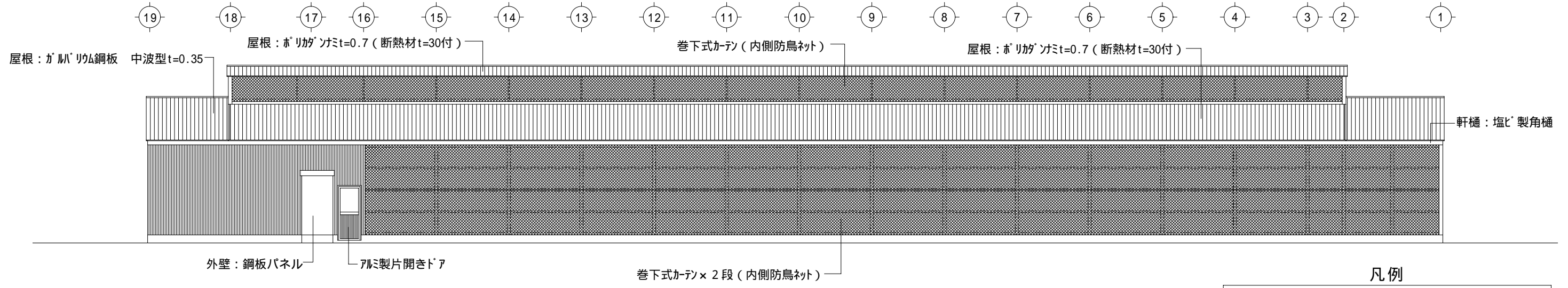
F 立面図 S=1/150
