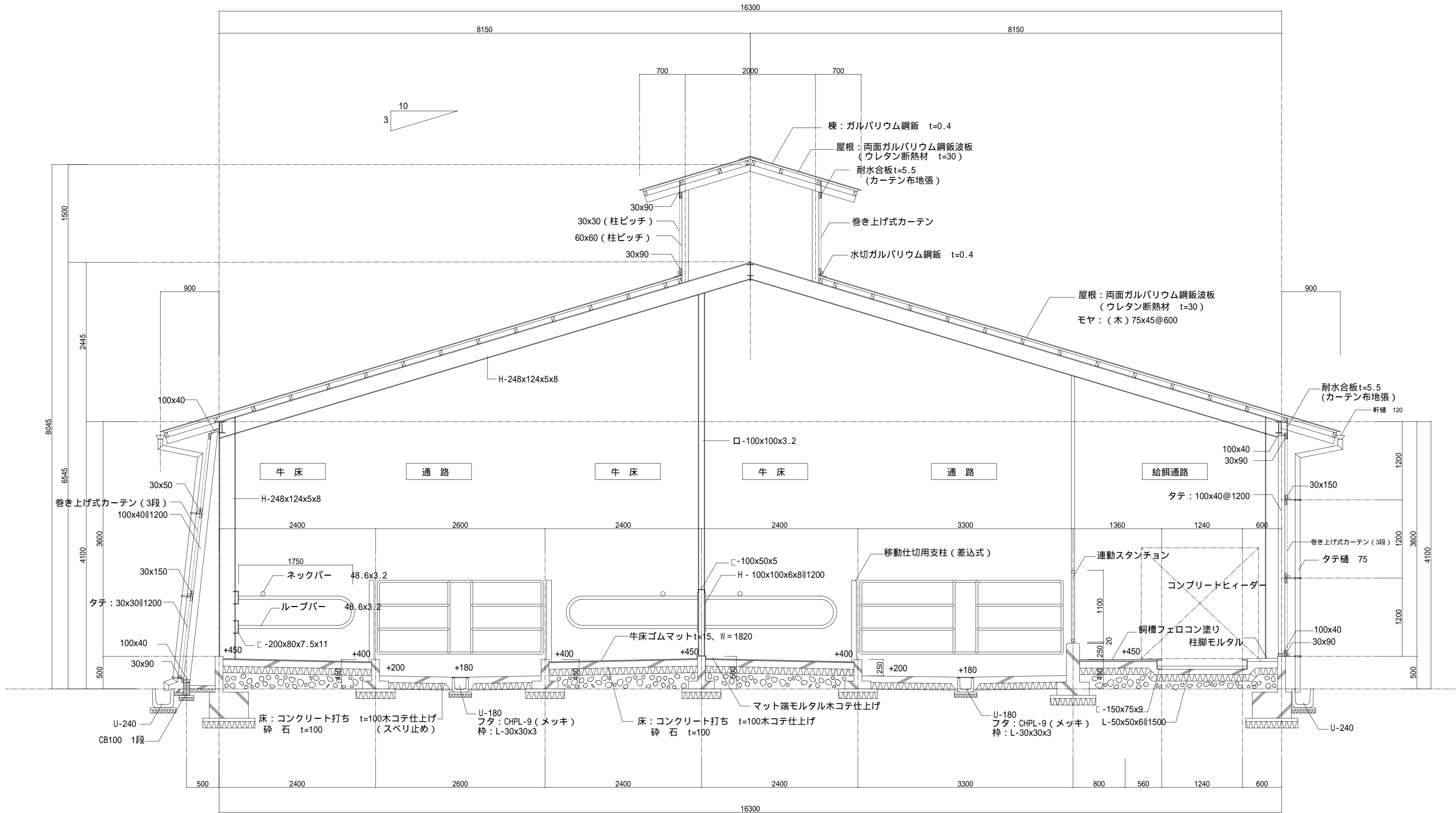
矩計図 S=1/40
