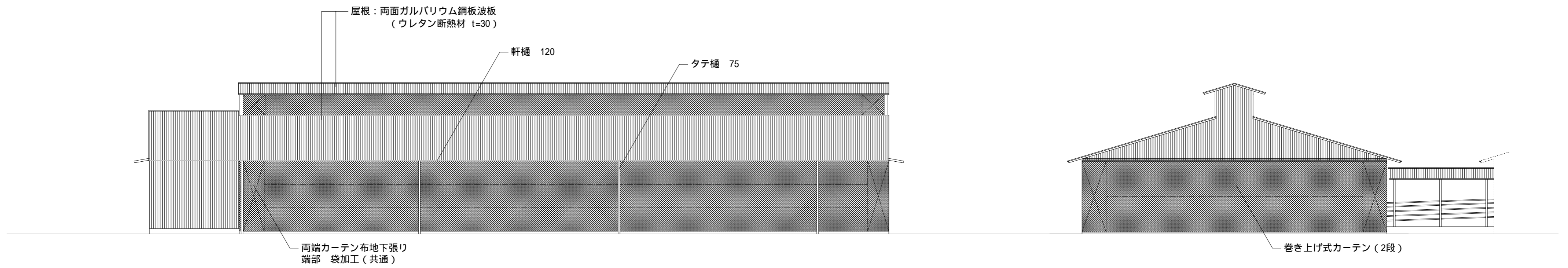
A通立面図 S=1/150
