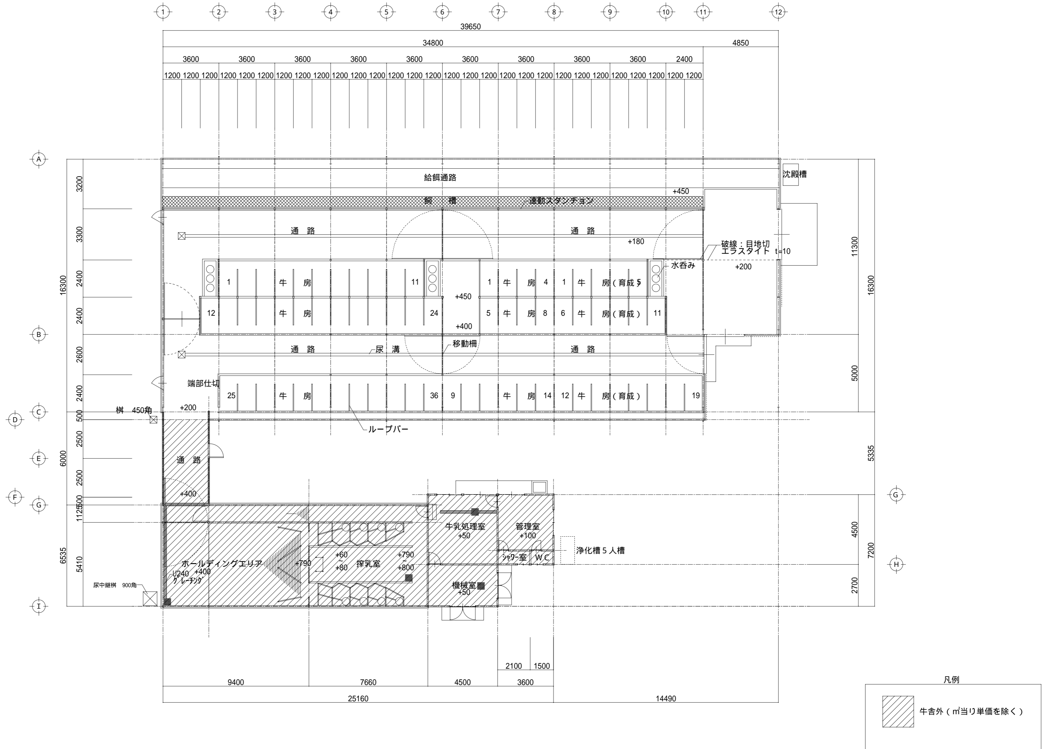
平面図 S=1/100
