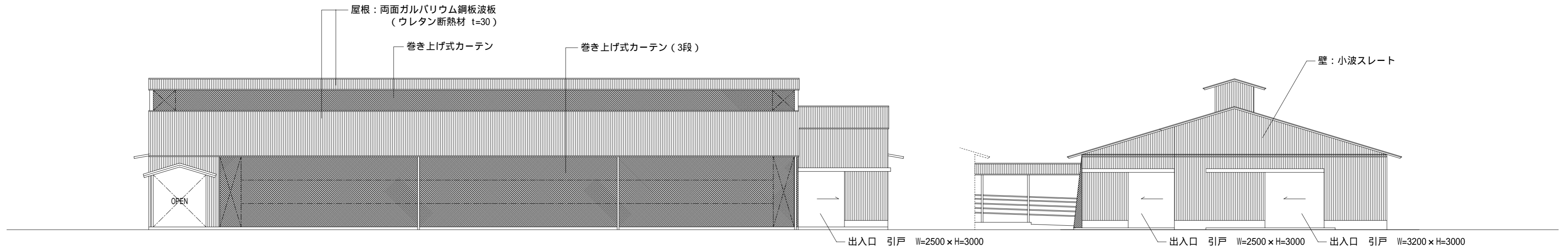
D通立面図 S=1/150
